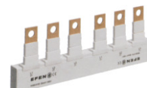
Einspeiseklemmen 052414 und 052419: für Set 3Stk. bestellen!
